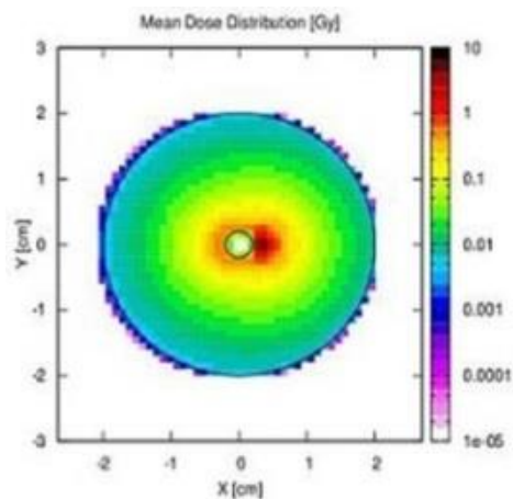
Рис. 5. Распределение поглощенной дозы в материале коллиматора в плоскости XY (Грей).
