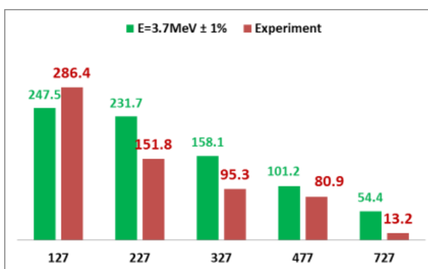
Рис. 18. Рассчитанная и измеренная мощность дозы в мкЗв/ч для различных позиций дозиметра прямого пучка, когда разброс первичной энергии составлял 0% (слева) и когда разброс энергии составлял 1% RMS (справа). Горизонтальная ось показывает расстояние от выхода электронной пушки в см.
