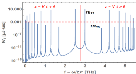
Рисунок 3: Спектральное распределение излучения дипольной моды ( n=1 ) в волноводе с медными стенками; излучение вперед (справа) и назад (слева).
