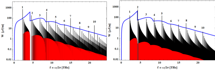
Рис. 1. Дискретный спектр излучения для ТМ (красные вертикальные линии) и ТЕ (черные вертикальные линии) мод в волноводе и в свободном пространстве (синий). Радиусы волновода b = 0.1m (слева) и 0.5m (справа), энергия частицы 15 МэВ, параметр ондулятора K=0,744 . Цифрами обозначен индекс n ( n = 1, 2, 3, \dots 10 ) TE_{n,m} мод волновода.
