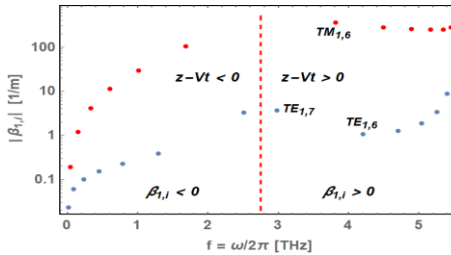
Рисунок 5: Коэффициенты затухания для ТЕ (синий) и ТМ (красный) мод на резонансных частотах при n=1 .
