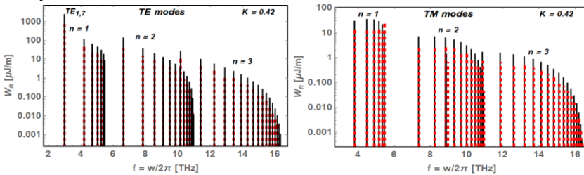
Рисунок 4: Спектральное распределение накопленной энергии излучения (пространственно-временная область, прямое направление, z - Vt \rightarrow 0_+ ) для первых трех мультиполей ( n=1,2,3 ) для ТЕ (слева) и ТМ (справа) мод в медном (красные пунктирные линии) и идеальном (черные сплошные линии) волноводах.
